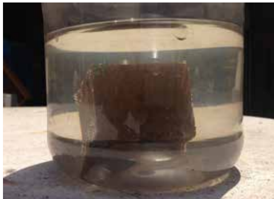
Figuras 7a y 7b. Probetas realizadas con tierra estabilizada con 6% de cal en peso seco y posteriormente compactadas por capas, han logrado subsistir su inmersión total en agua por más de 10 años. (Foto: L. Guerrero).
